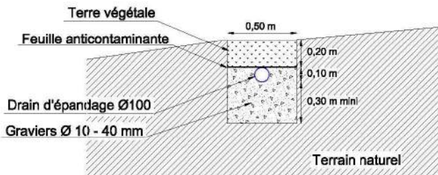
Tranchées d'épandage Profonde
