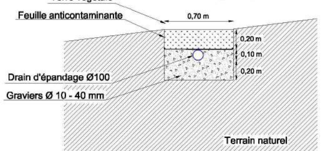
Tranchées d'épandage Large
