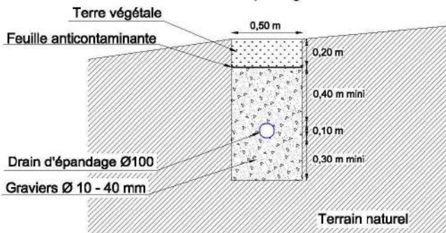
Tranchées d'épandage Profonde
